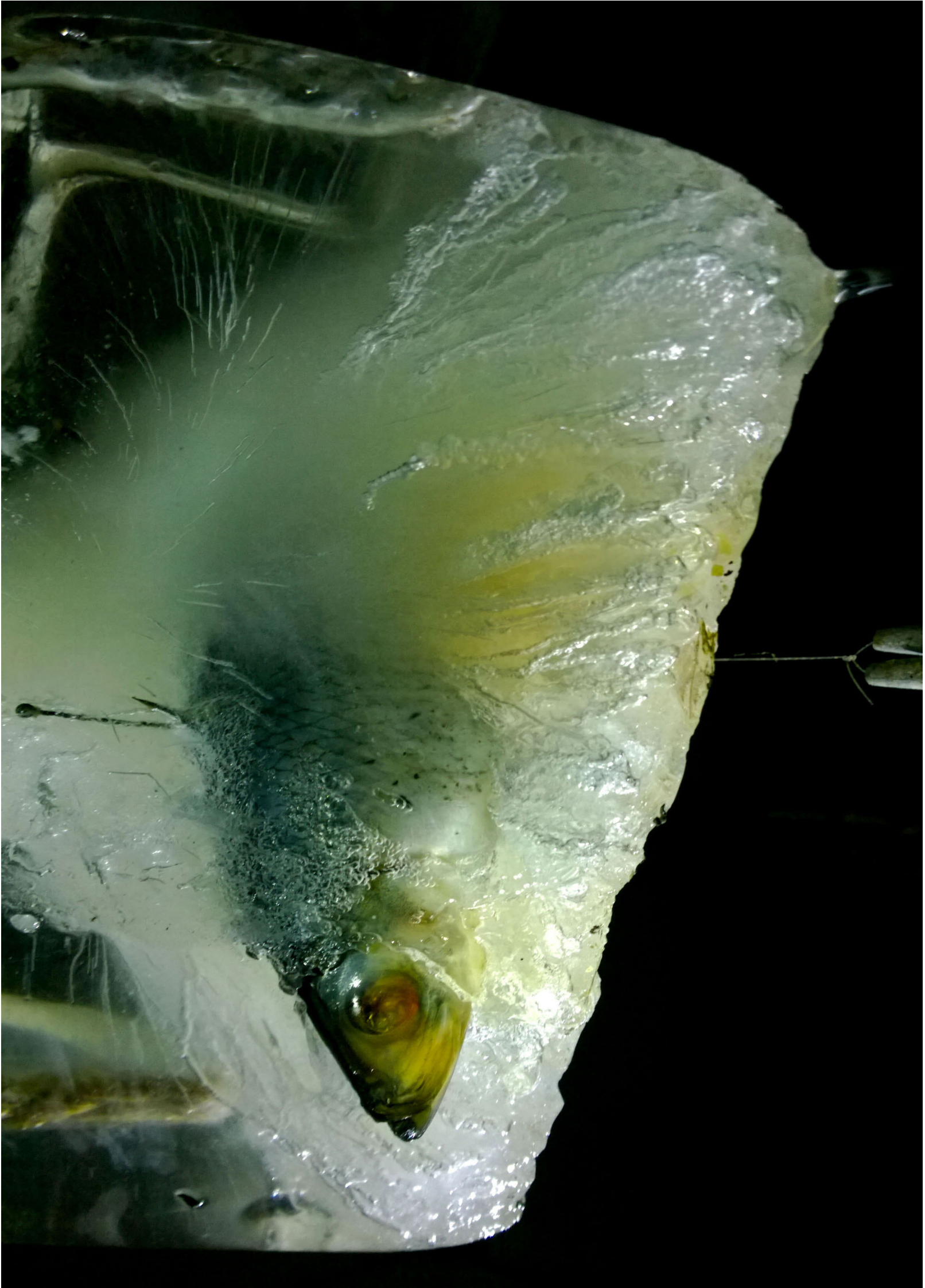
magnitude 2.0
